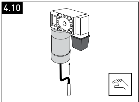
Umieścić korbę bezpośrednio w napędzie.
