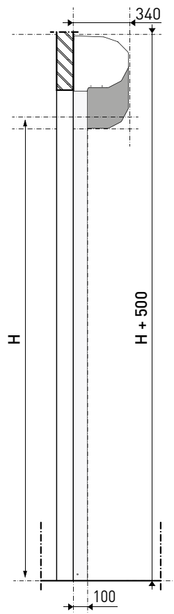
[ Przekrój poprzeczny ]
