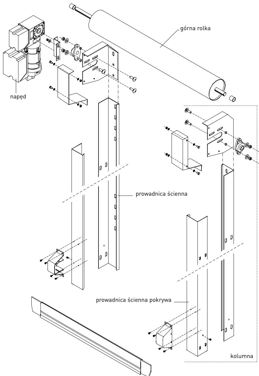
Rysunek złożeniowy
